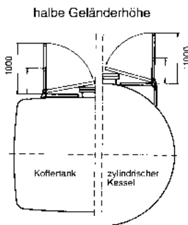
Seitlich klappbares Geländer
